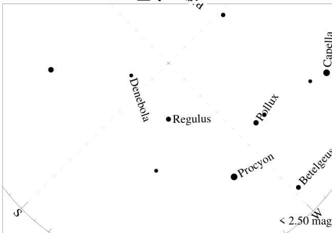
星等 2 级
