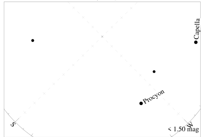
星等 1 级
