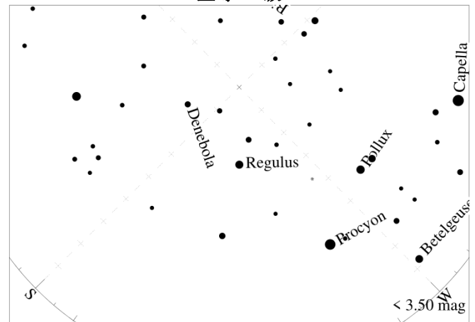
星等 3 级
