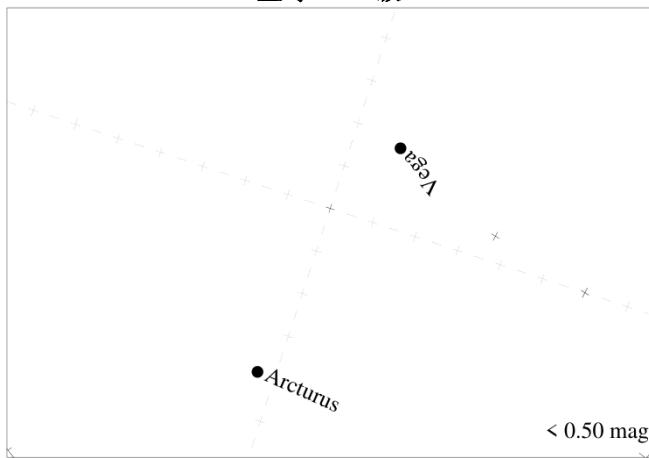
星等 < 1 级
