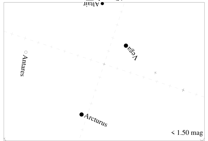
星等 1 级
