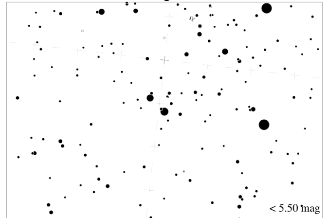
Carte Magnitude 5
