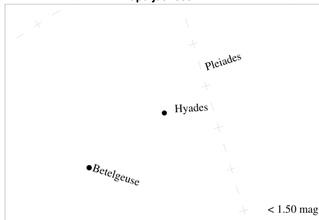
Mapa jasności 1
