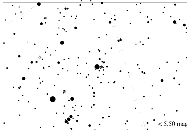
Mapa jasności 5
