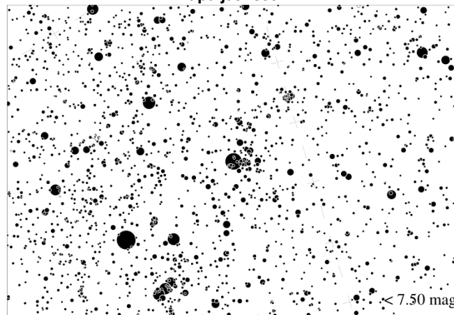
Mapa jasności 7
