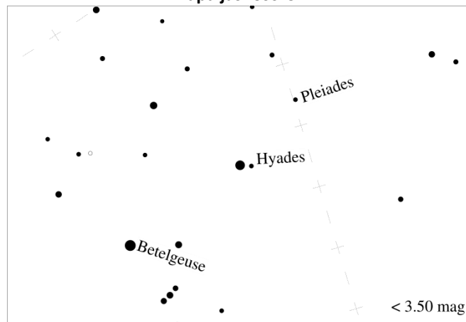
Mapa jasności 3
