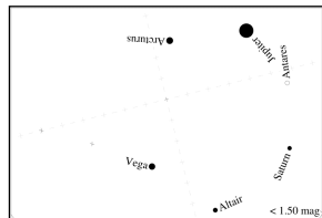
Карта звезда 1. магнитуде
