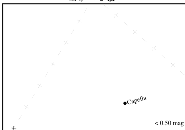
星等 < 1 级
