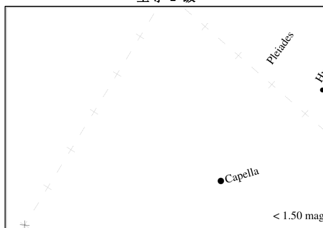
星等 1 级
