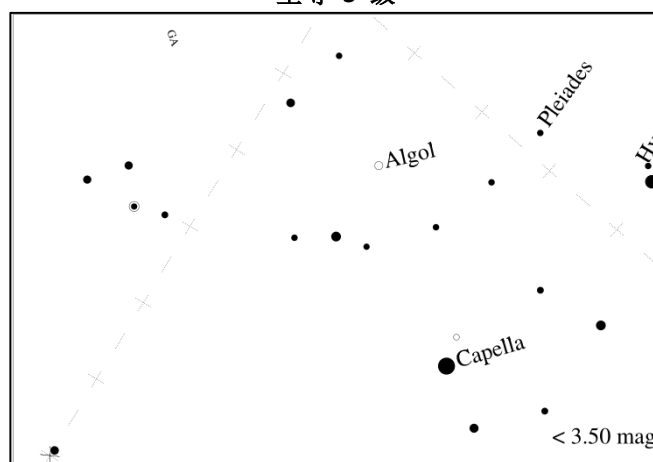
星等 3 级
