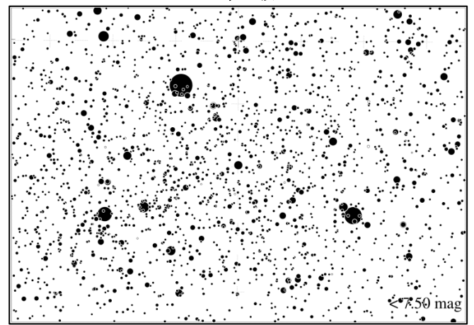
星等 7 级
