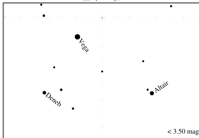
星等 3 级
