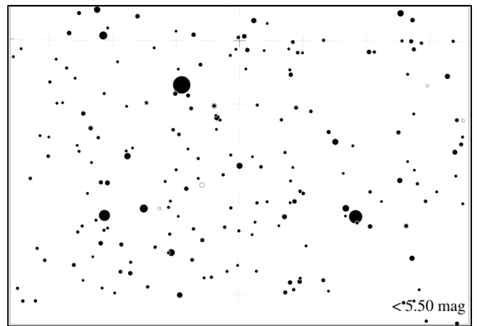
星等 5 级
