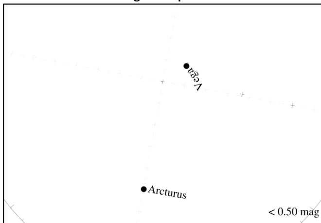
Magnitúda pod 1
