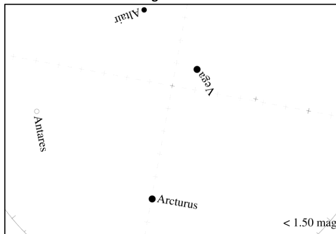
Magnitúda 1
