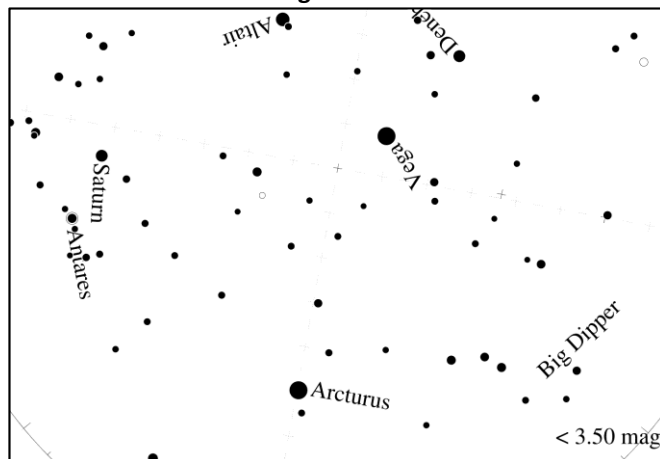
Magnitúda 3
