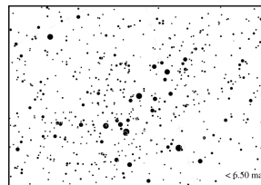
Peta Magnitudo 6
