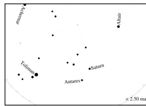
Peta Magnitudo 2
