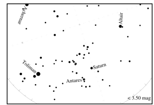
Peta Magnitudo 3
