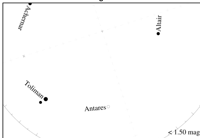
Peta Magnitudo 1
