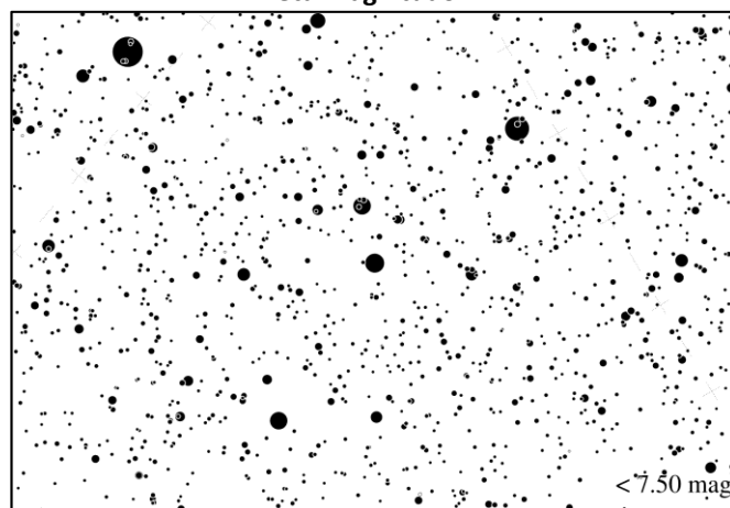
Peta Magnitudo 7
