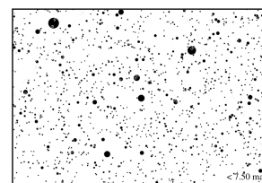
Peta Magnitudo 7
