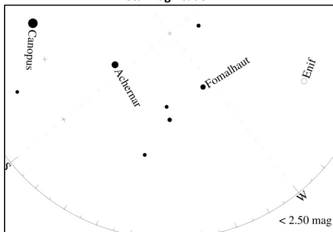
Peta Magnitudo 2
