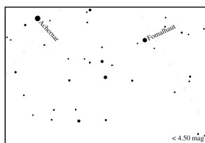
Peta Magnitudo 4
