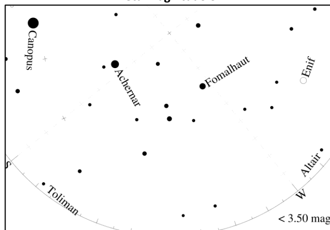
Peta Magnitudo 3
