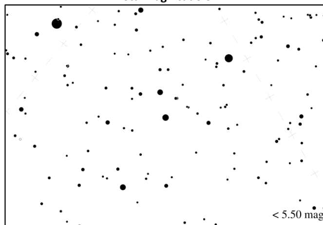
Peta Magnitudo 5
