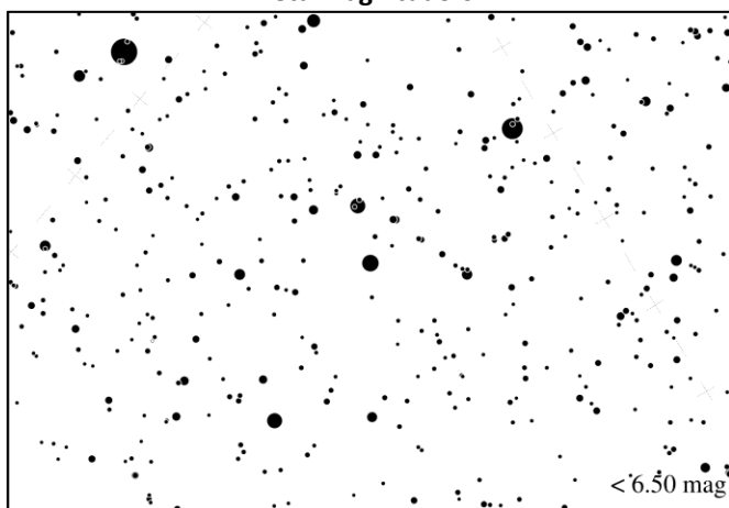
Peta Magnitudo 6
