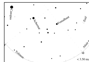
Peta Magnitudo 3
