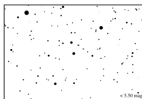
Peta Magnitudo 5
