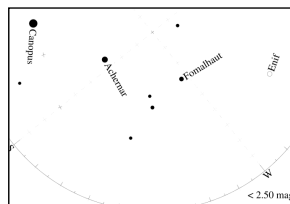
Peta Magnitudo 2
