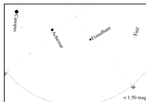
Peta Magnitudo 1
