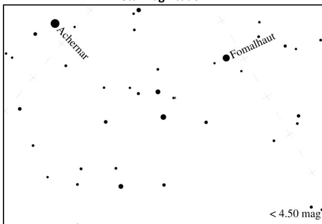
Peta Magnitudo 4
