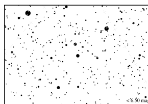
Peta Magnitudo 6
