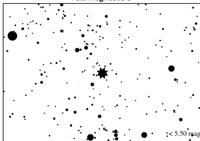
Peta Magnitudo 5
