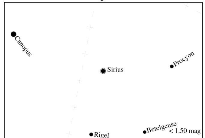
Peta Magnitudo 1
