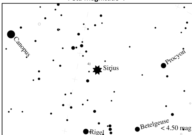
Peta Magnitudo 4
