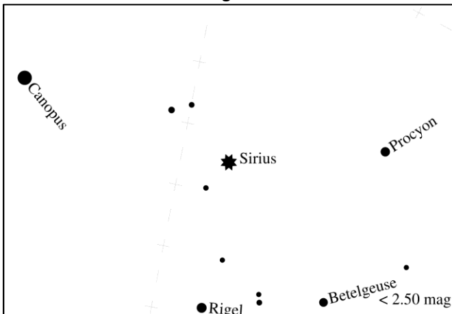
Peta Magnitudo 2
