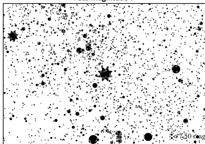
Peta Magnitudo 7
