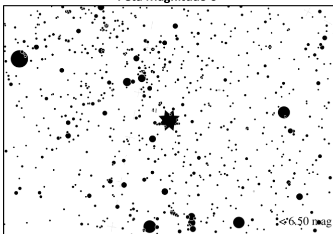
Peta Magnitudo 6
