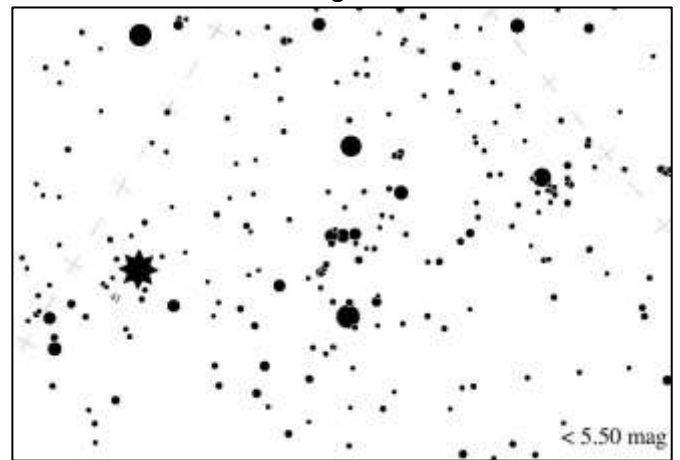
Peta Magnitudo 5
