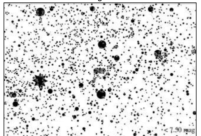
Peta Magnitudo 7
