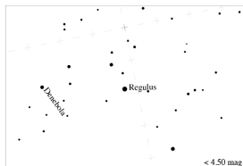
星図4
