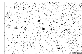
星図7
