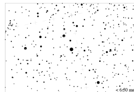
星図6
