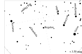
星図3
