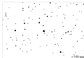
星図5
