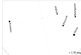
星図1
