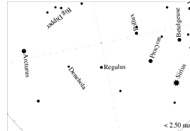
星図2
