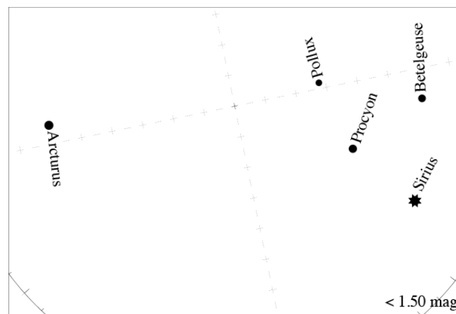
星図1
