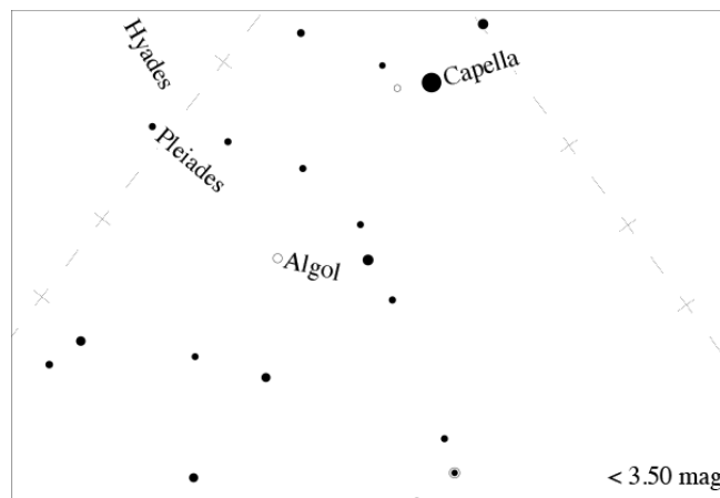
星図3
