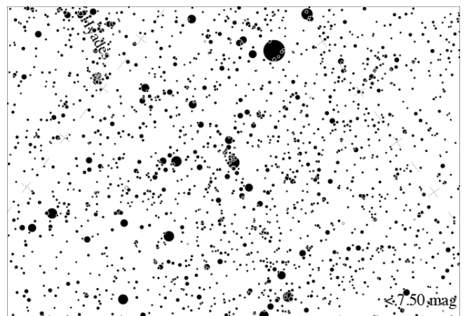
星図7
