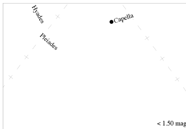
星図1
