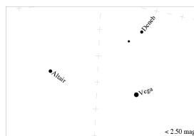
OMapa jasności 2
