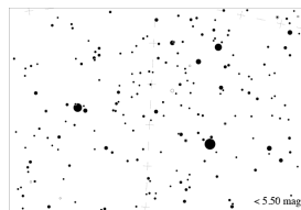
OMapa jasności 5
