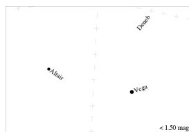
OMapa jasności 1
