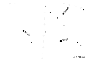
OMapa jasności 3
