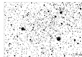
OMapa jasności 7
