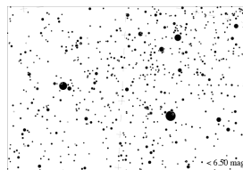
OMapa jasności 6
