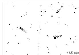
OMapa jasności 4
